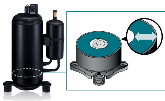
Sprężarka
